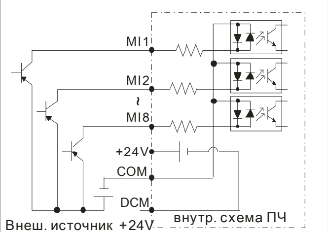
④ PNP-режим с внешним питанием
